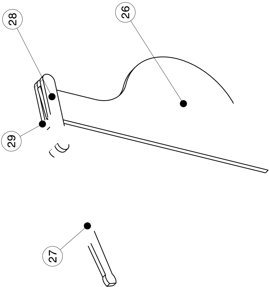
F Rudder Assy Scale: 1:8
